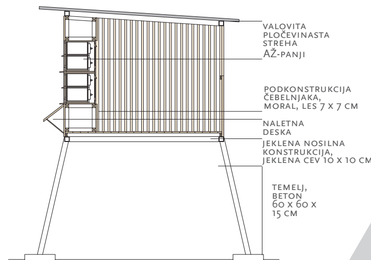
VZDOLŽNI PREREZ
