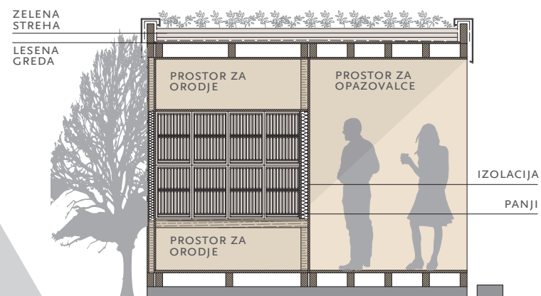
PREREZ BB
