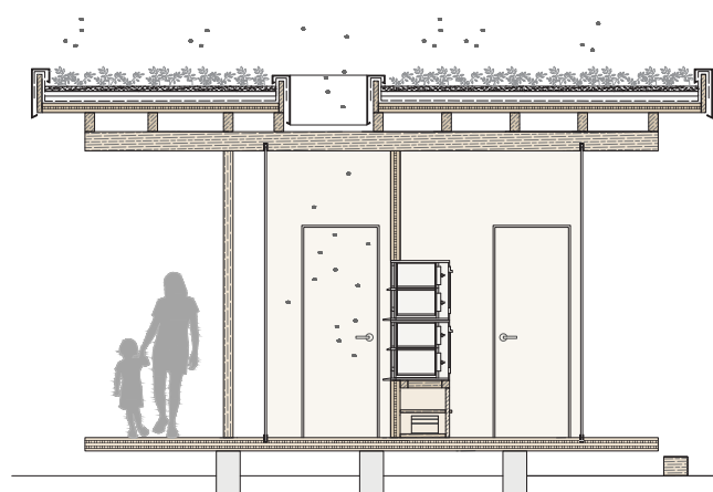
PREREZ
